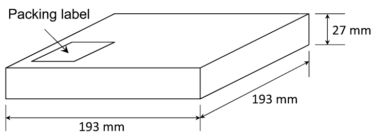
Fig. 16.4.1 1 reel/carton
